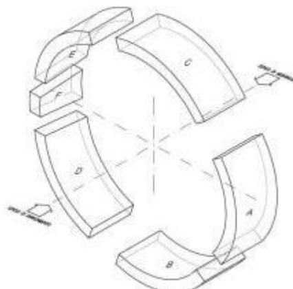
Figura 3-12. Exemplu de reprezentare axonometrică a inelului cu dispunerea segmentului
