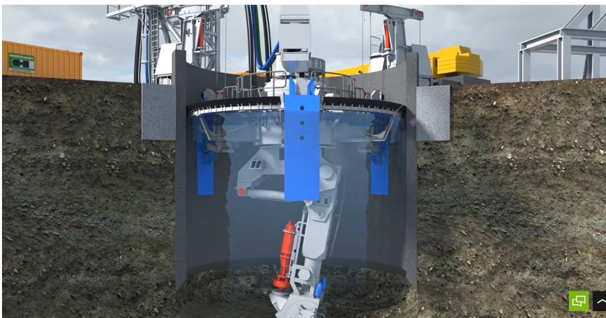
Figura 3-18. Exemplu pentru mașina de realizare a putului vertical
