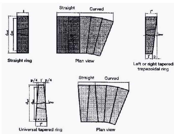
Figura 3-9. Dispunerea inelelor drepte și conice pentru secțiuni drepte și curbate
