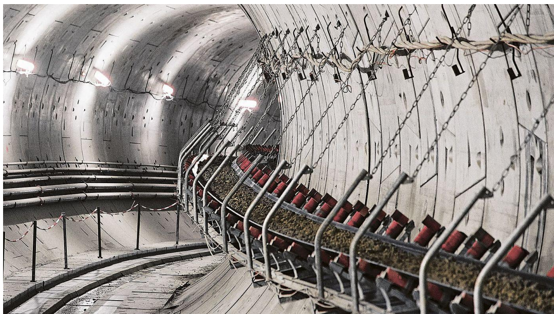
Figura 10-8.: Transportor cu bandă pentru material excavat în interiorul tunelului
