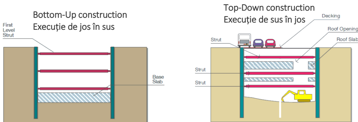
Figura 3-3. Metoda de săpătură deschisă: construcție convențională de jos în sus (stânga) și construcție de sus în jos (dreapta)
