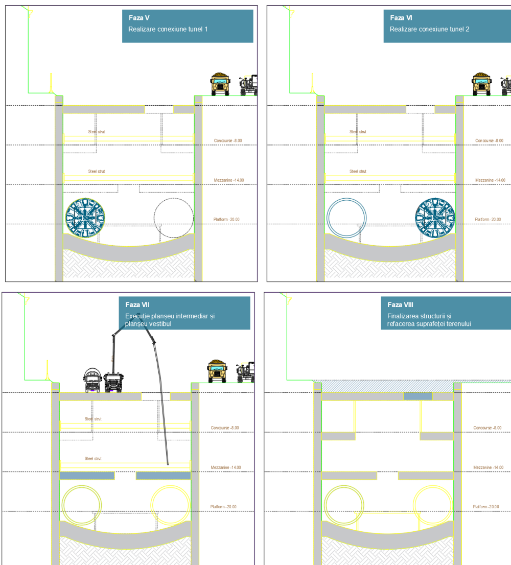
Figura 3-2. Tehnologie de execuție top-down
