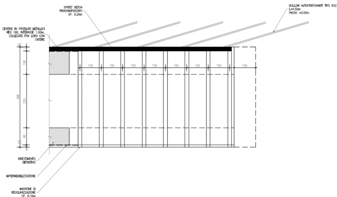
Figura 3-17. Consolidare temporară pentru tunelul orizontal
