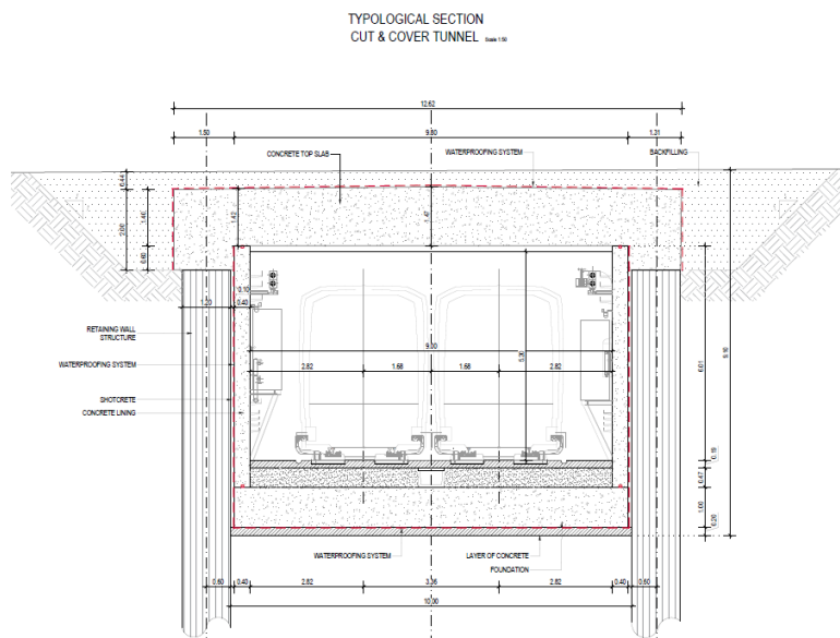
Figura 3-4. Secțiune tip Metoda Cut & Cover – Săpătură deschisă
