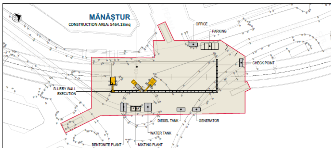
Figura 10-2.: Organizarea de șantier Stația Mănăștur
