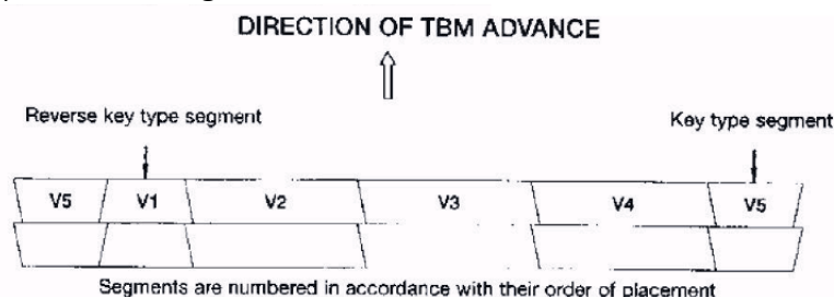
Figura 3-11. Distribuția tipică a paralelogramelor și a segmentelor trapezoidale pentru inelele de căptușire
