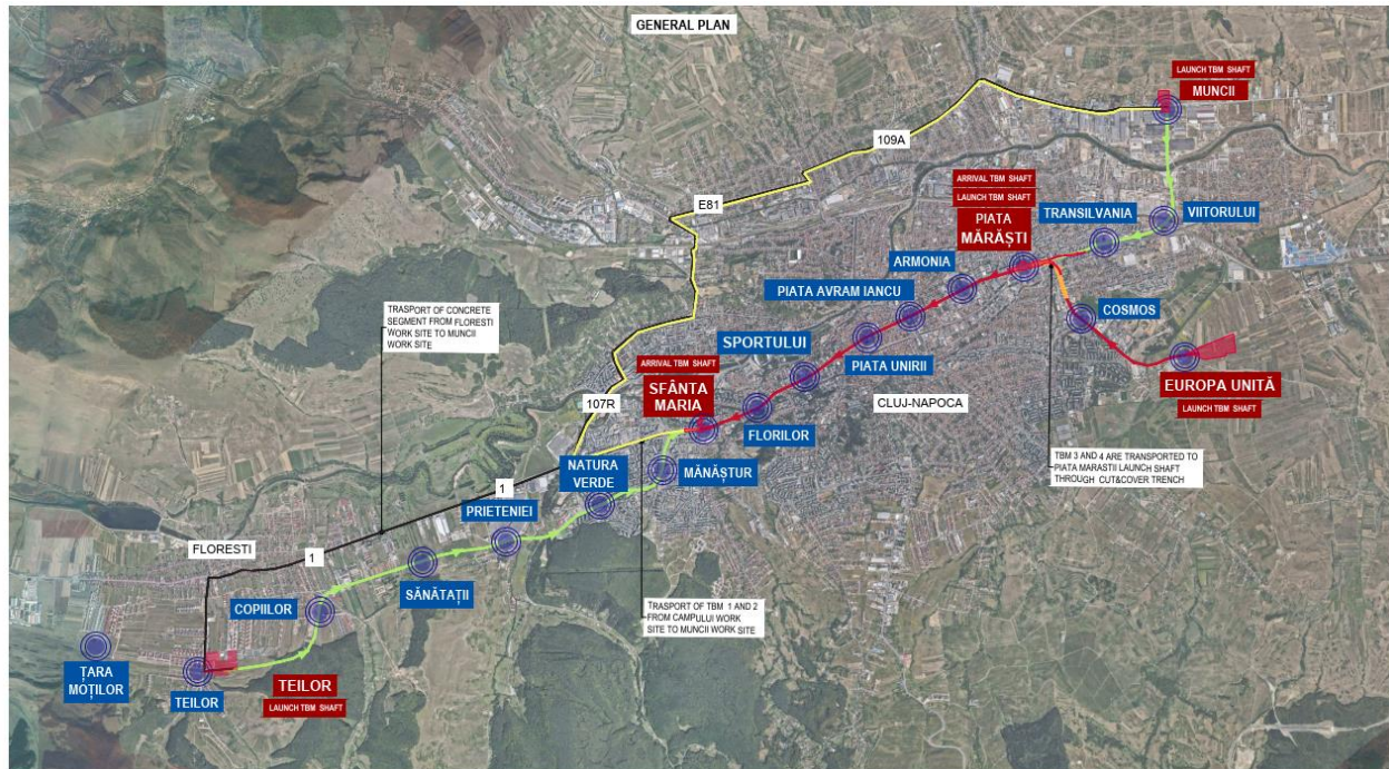
Figura 10-3.: Plan general pentru amplasarea organizărilor de șantier
