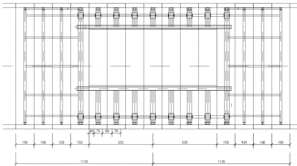
Figura 3-15. Cadru de armare din oțel în corespondență cu tăierea segmentelor de căptușeală a tunelului de metrou
