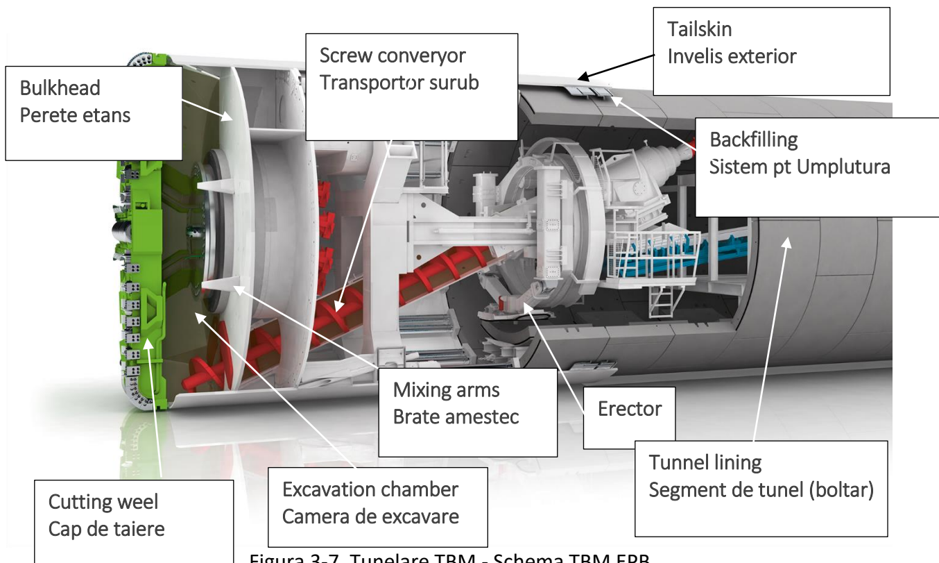
Figura 3-7. Tunelare TBM - Schema TBM EPB
