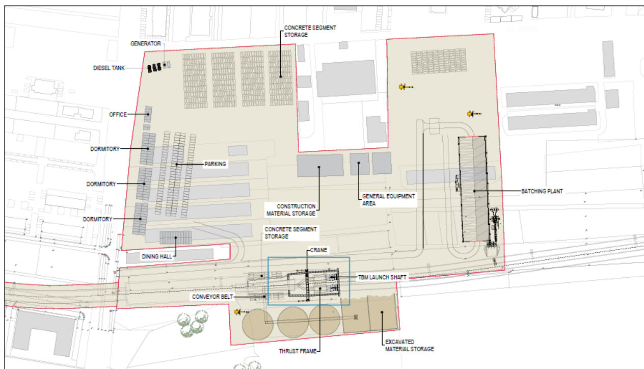
Figura 10-12. Organizarea de șantier pentru TBM de la Stația Teilor
