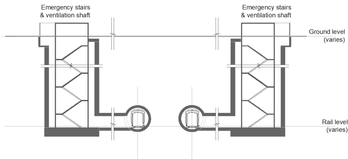
Figura 3-13. Secțiune transversală pentru ieșire de urgență verticală
