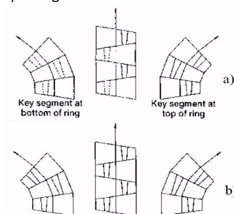
Figura 3-10. Utilizarea inelelor dreapta și stânga (a) și a inelelor universale (b) pentru secțiuni drepte și curbate
