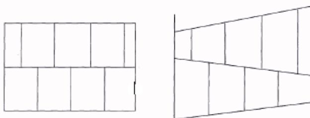
Figura 3-8. Tip de segment - Inele drepte (stânga), inele conice (dreapta)
