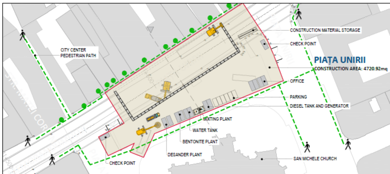
Figura 10-1.: Organizarea de șantier Stația Piața Unirii
