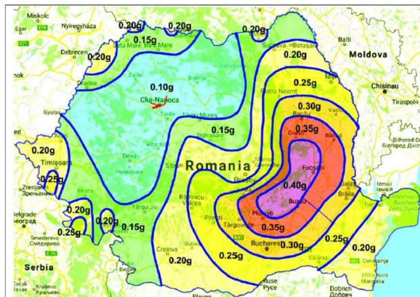
Figura 15-5. Zonarea valorilor de varf ale accelerației terenului pentru proiectare
