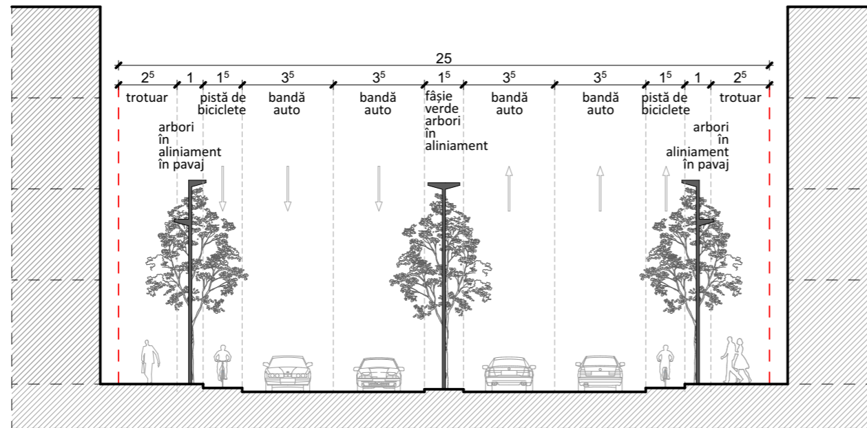
PROFIL TRANSVERSAL
