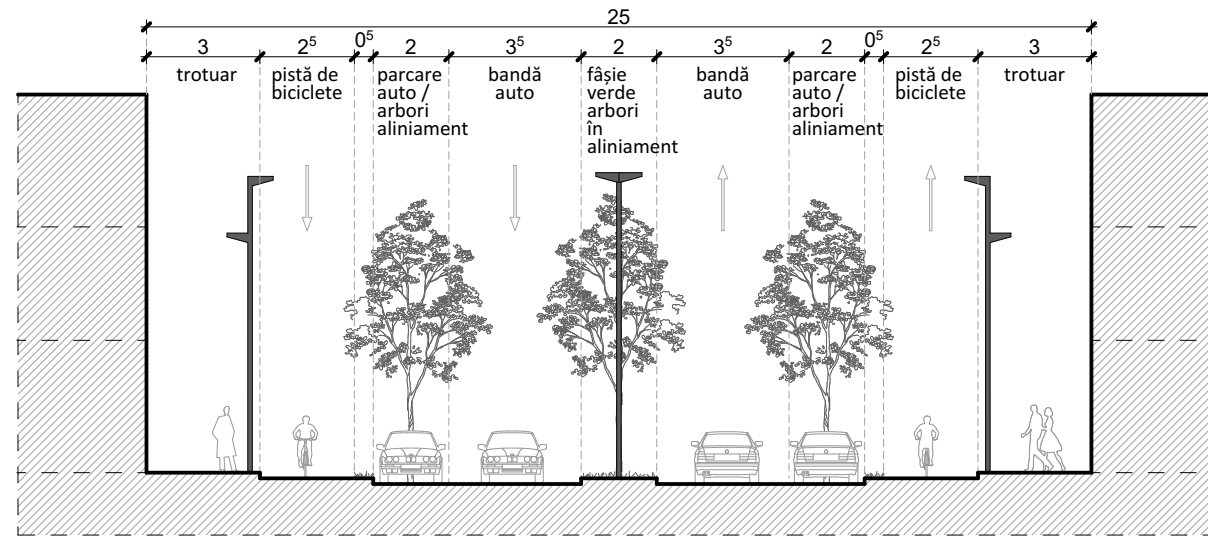
PROFIL TRANSVERSAL
