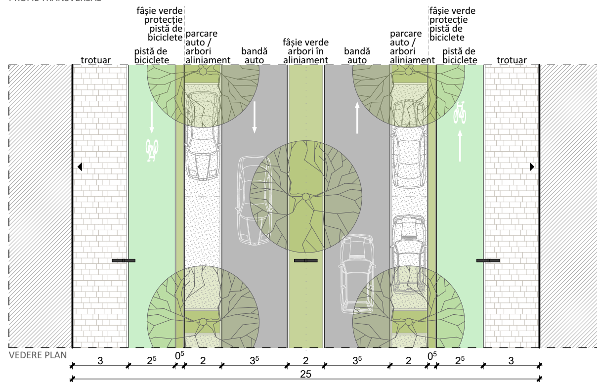
PROFIL TRANSVERSAL
