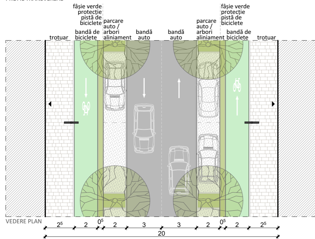
PROFIL TRANSVERSAL
