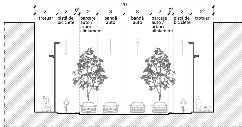
PROFIL TRANSVERSAL
