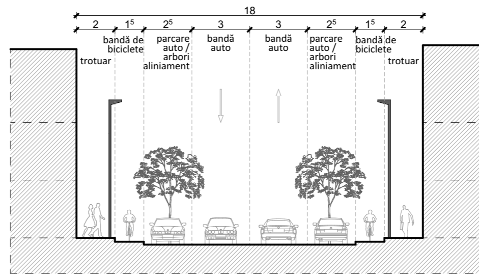
PROFIL TRANSVERSAL
