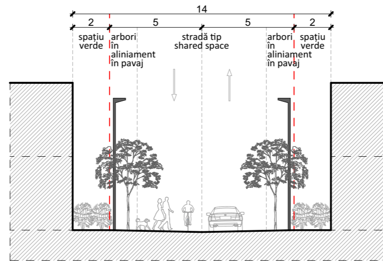
PROFIL TRANSVERSAL
