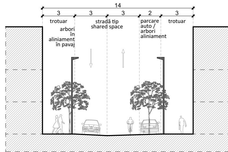
PROFIL TRANSVERSAL
