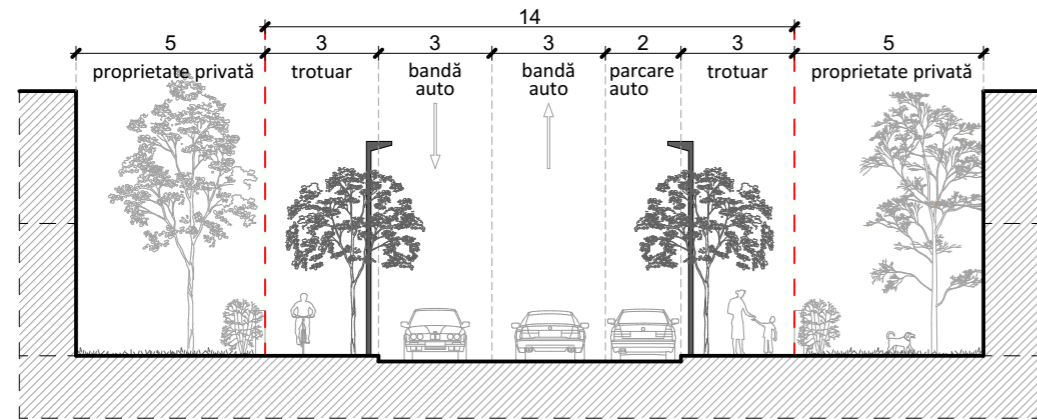
PROFIL TRANSVERSAL
