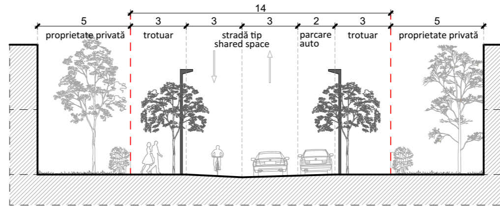
PROFIL TRANSVERSAL
