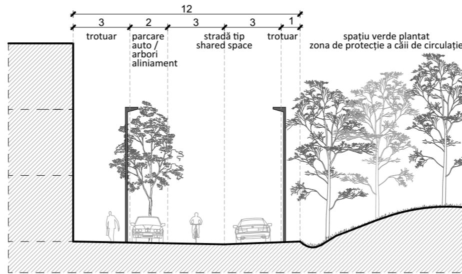
PROFIL TRANSVERSAL
