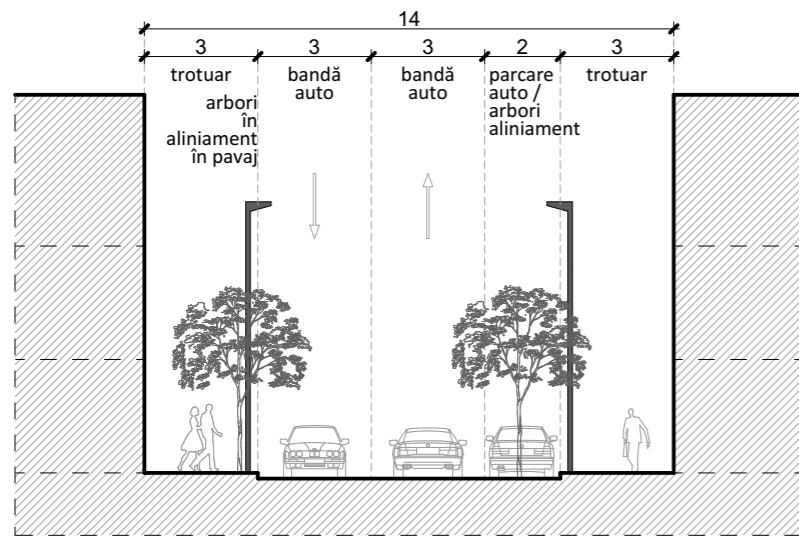
PROFIL TRANSVERSAL
