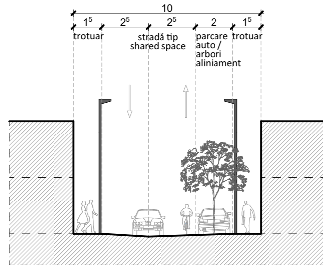
PROFIL TRANSVERSAL
